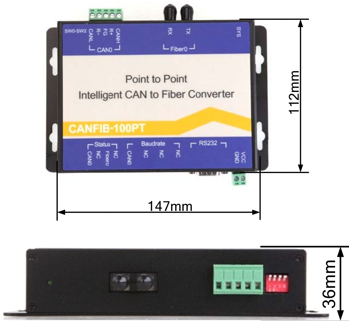
图 2-1-1 CANFIB-100PT 智能CAN光纤转换器机械尺寸
