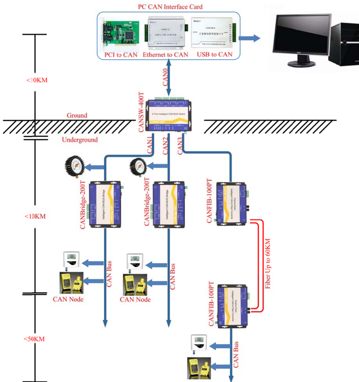
图 1-1-2 系列产品典型应用
