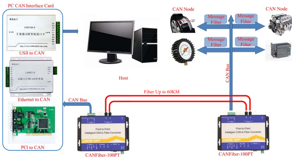
图 1-1-1 CANFIB-100PT 智能CAN光纤转换器典型应用
